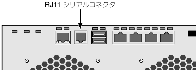
図 24. シリアルコネクタは、コントローラに位置しています
