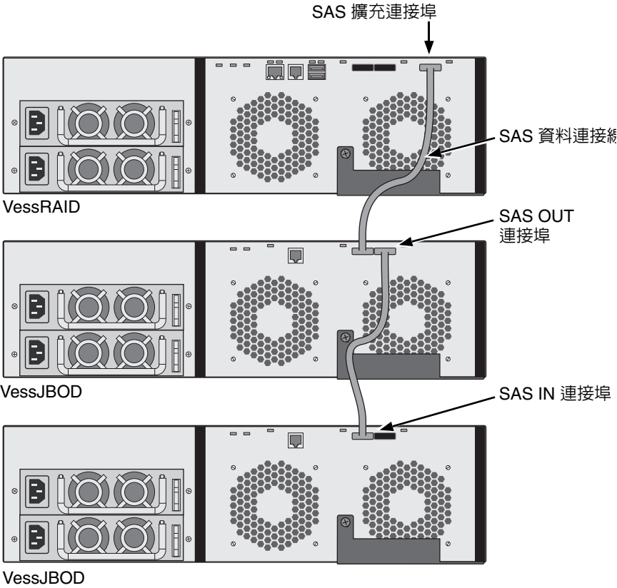
圖 23. SAS JBOD 擴充資料連接
