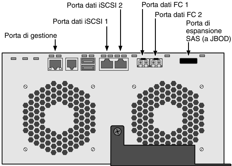
Figura 16. Collegamenti dati e gestione DAS FC
