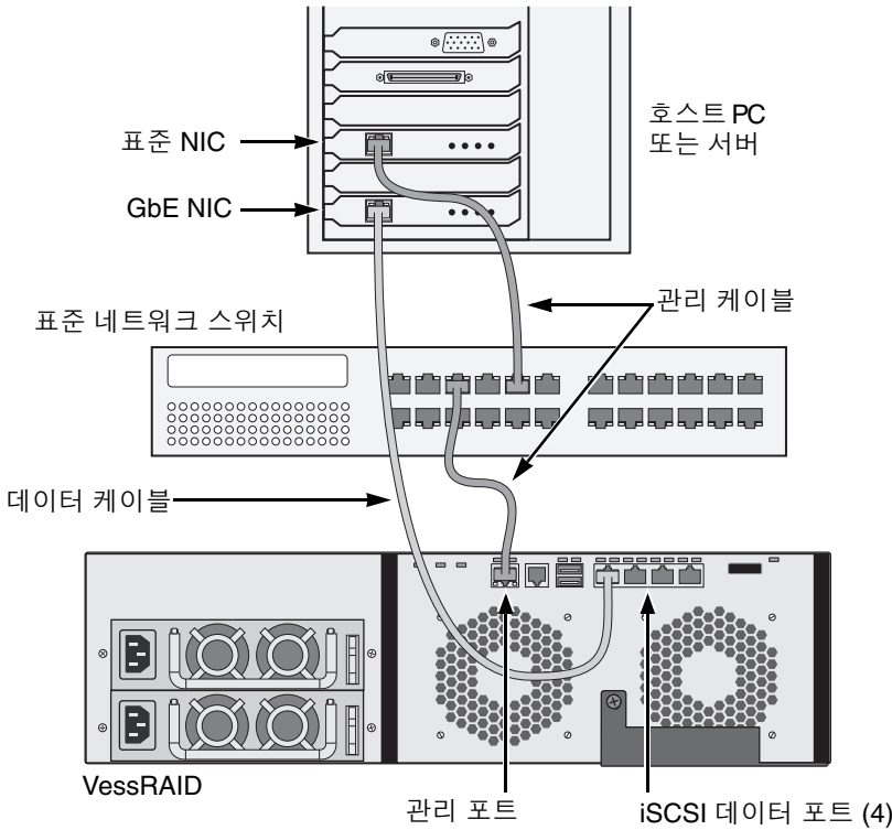
그림 19. iSCSI DAS 데이터 및 관리 커넥션
