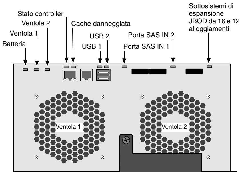
Figura 28. LED del controller SAS del VessRAID
