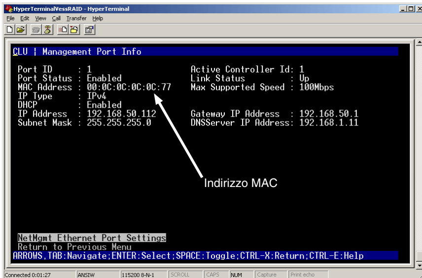
Figura 31. Visualizzazione dell'indirizzo MAC della porta di gestione.
