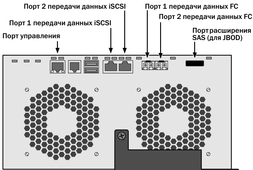
Рис. 15. Порты передачи данных и управления FC устройства VessRAID
