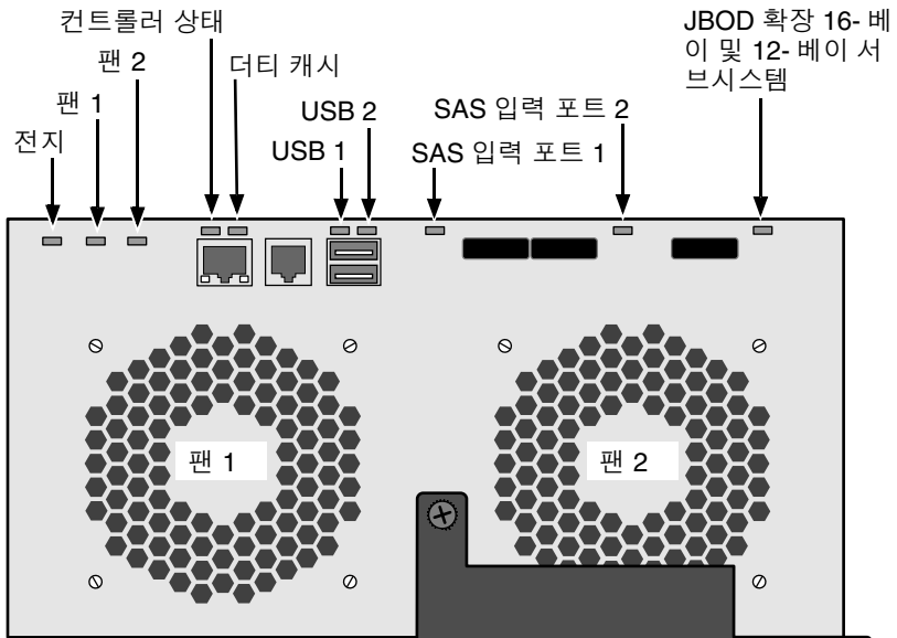
그림 28. VessRAID SAS 컨트롤러 LEDs
