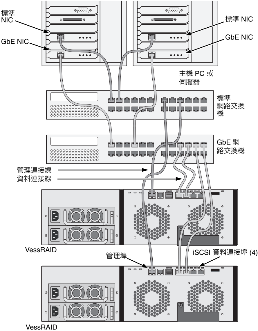
圖 20. iSCSI SAN 資料與管理連接
