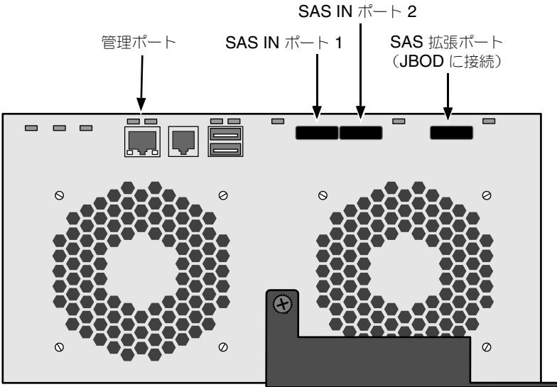
図 22. SAS DAS データおよび管理接続
