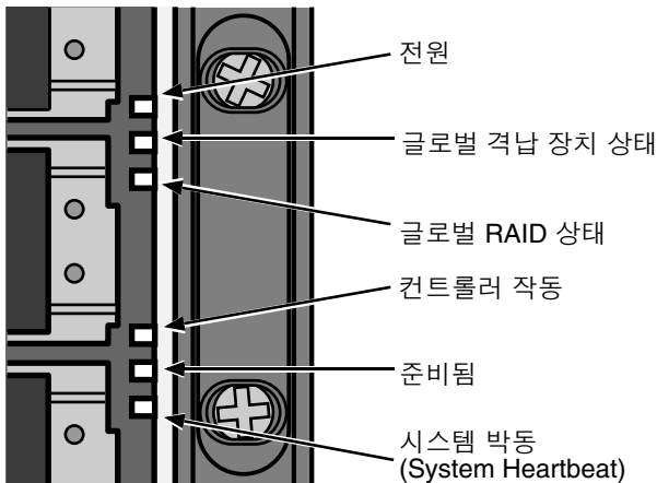
그림 25. VessRAID 전면 패널 LED 디스플레이
