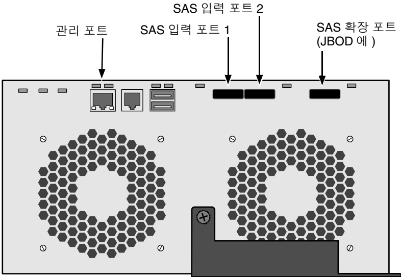
그림 22. SAS DAS 데이터 및 관리 연결
