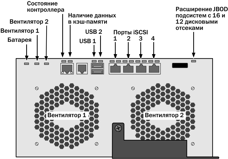
Рис. 27. Индикаторы контроллера VessRAID iSCSI
