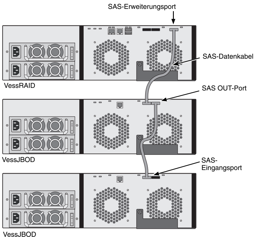
Abbildung 23. SAS JBOD-Erweiterungsdatenanschlüsse
