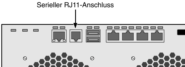
Abbildung 24. Ein serieller Anschluss ist auf dem Controller vorhanden
