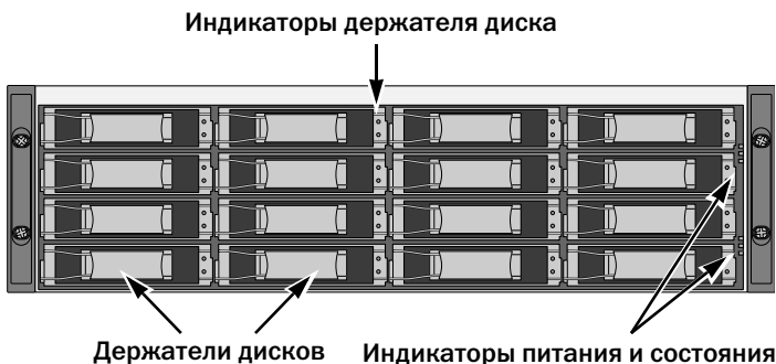
Рис. 1. Вид спереди устройства VessRAID с 16 дисковыми отсеками
