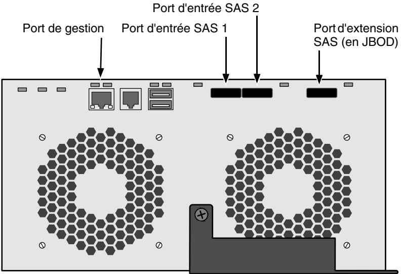
Figure 22. Connexions de gestion et de données SAS DAS
