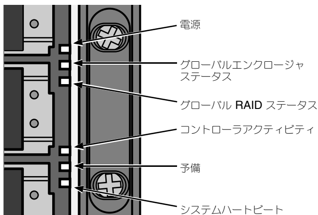
図 25. VessRAID の前面パネルの LED 表示
