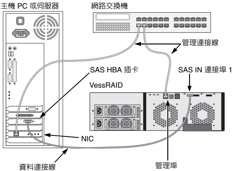
圖 22. SAS DAS 資料與管理連接
