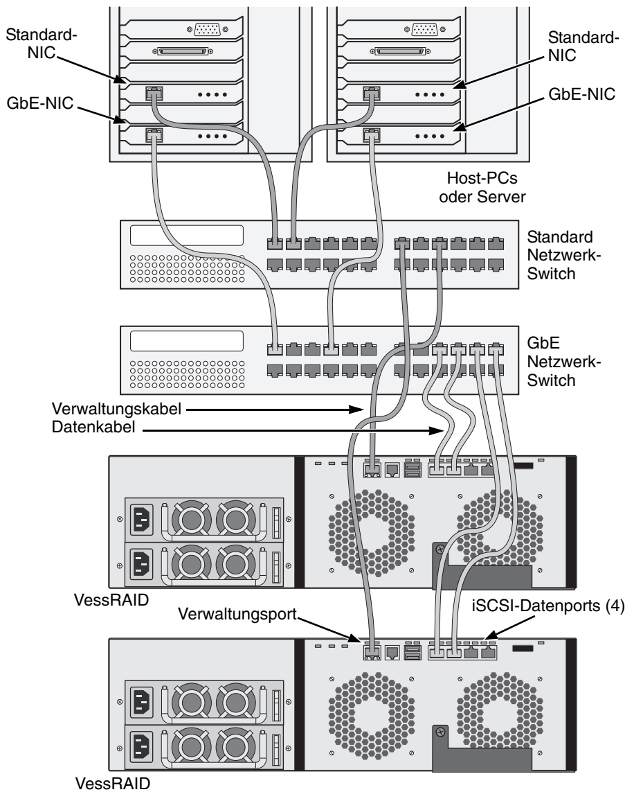
Abbildung 20. iSCSI SAN-Daten und Verwaltungsanschlüsse
