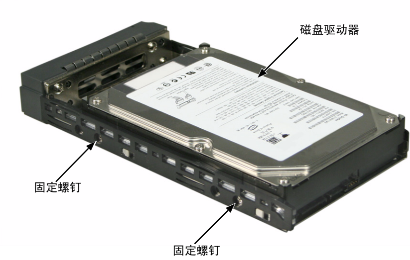
图 14。安装在驱动器托架中的磁盘驱动器
