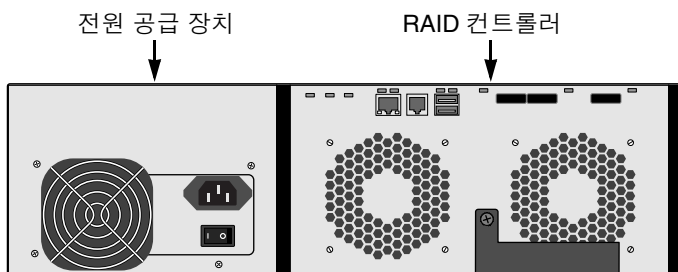
그림 6. VessRAID 1740s 후면 모습
