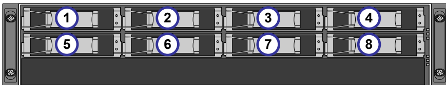
图 13。8 托架 VessRAID 驱动器插槽编号
