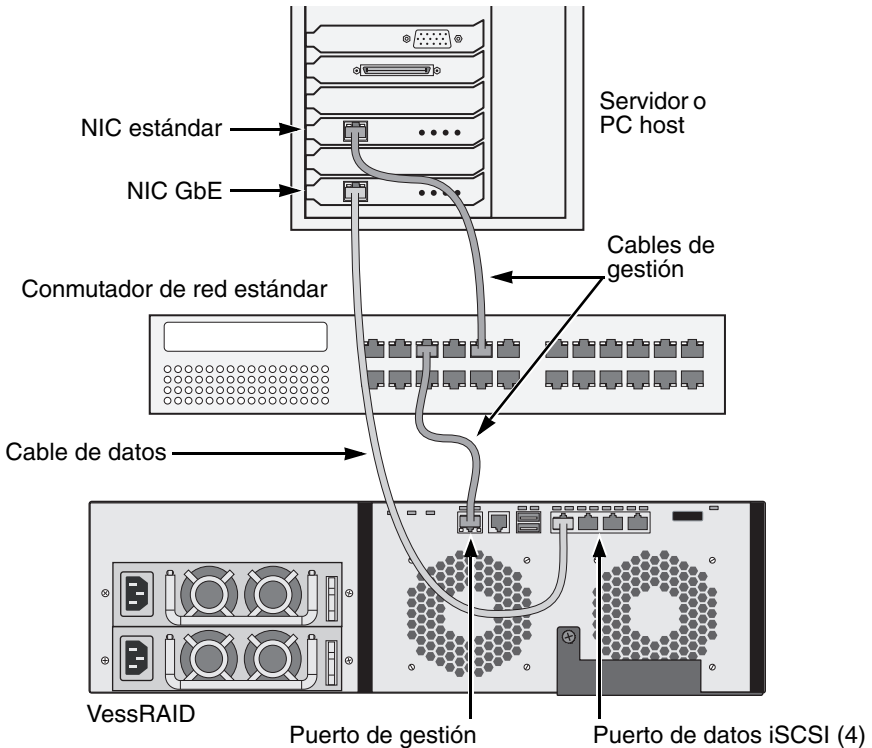
Ilustración 19. Conexiones de gestión y datos de DAS iSCSI
