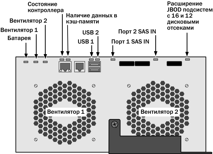
Рис. 28. Индикаторы контроллера VessRAID SAS
