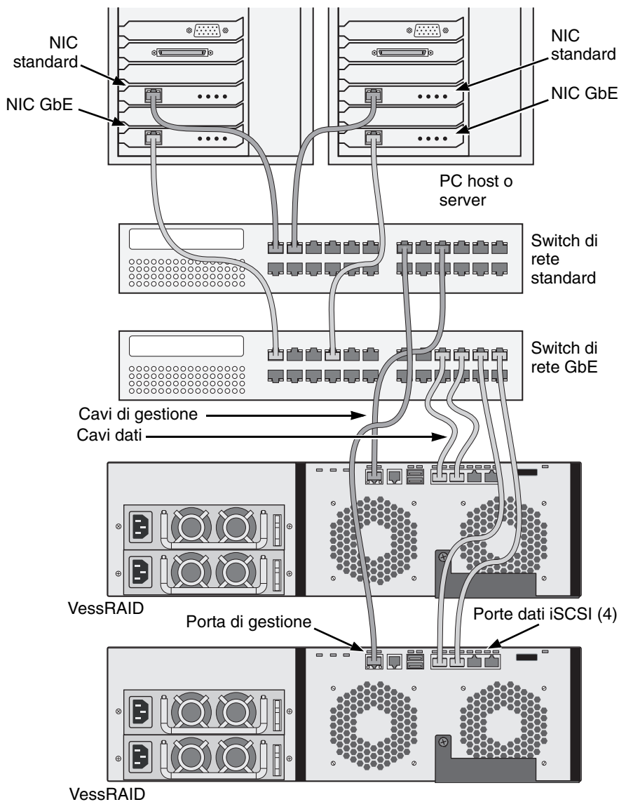
Figura 20. Collegamenti dati e gestione SAN iSCSI
