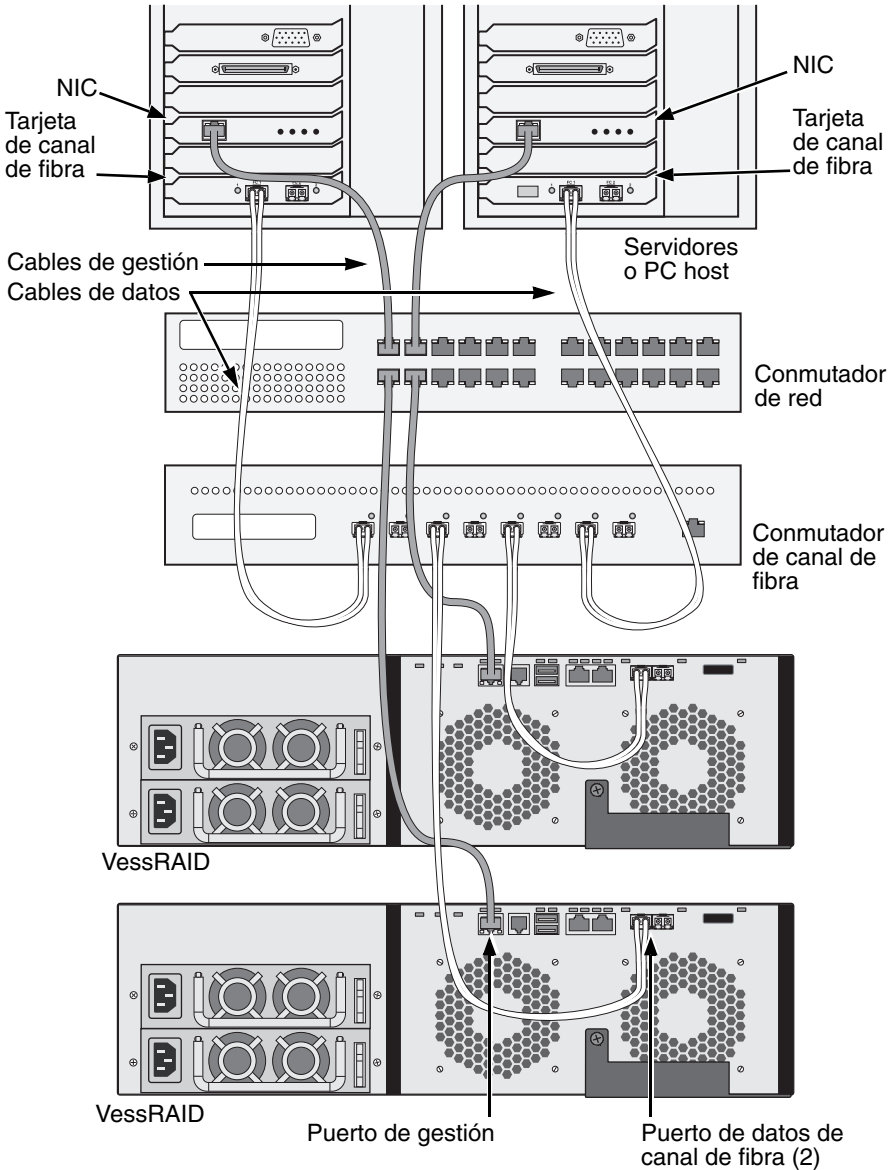
Ilustración 17. Conexiones de gestión y datos de SAN de canal de fibra
