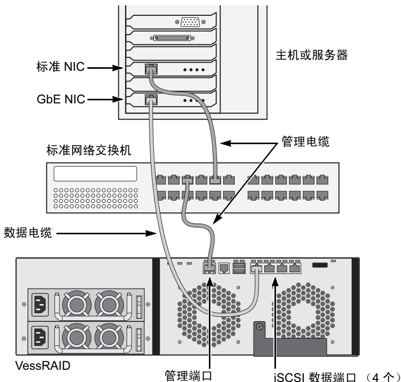
图 19。iSCSI DAS 数据和管理连接
