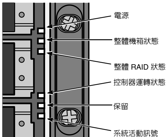
圖 25. VessRAID 前面板 LED 顯示器
