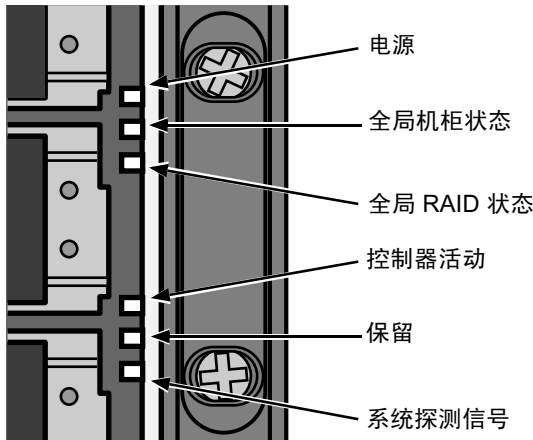
图 25。VessRAID 前面板 LED 指示灯显示
