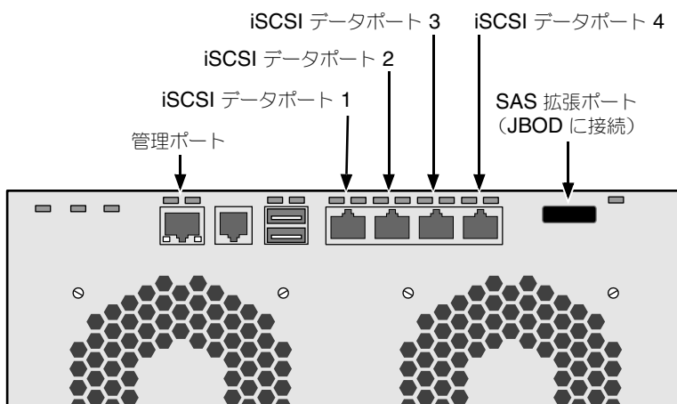
図 19. iSCSI DAS データおよび管理接続
