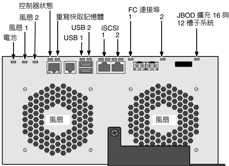
圖 26. VessRAID FC 控制器 LED
