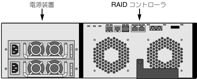
図 3. VessRAID 1840i 背面図
