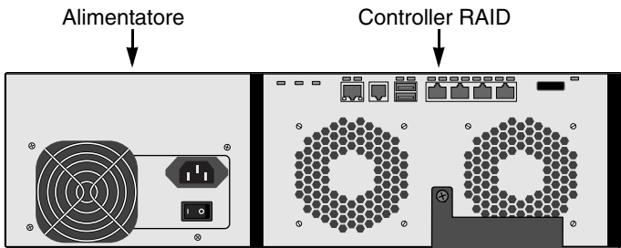
Figura 5. Vista posteriore del VessRAID 1740i
