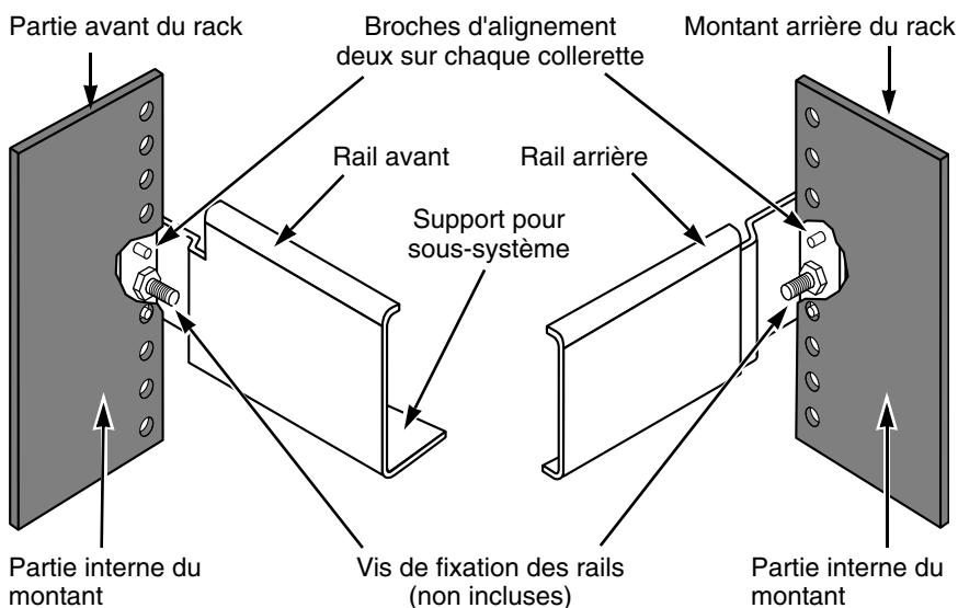
Figure 10. Schéma d'assemblage pour le montage du rack
