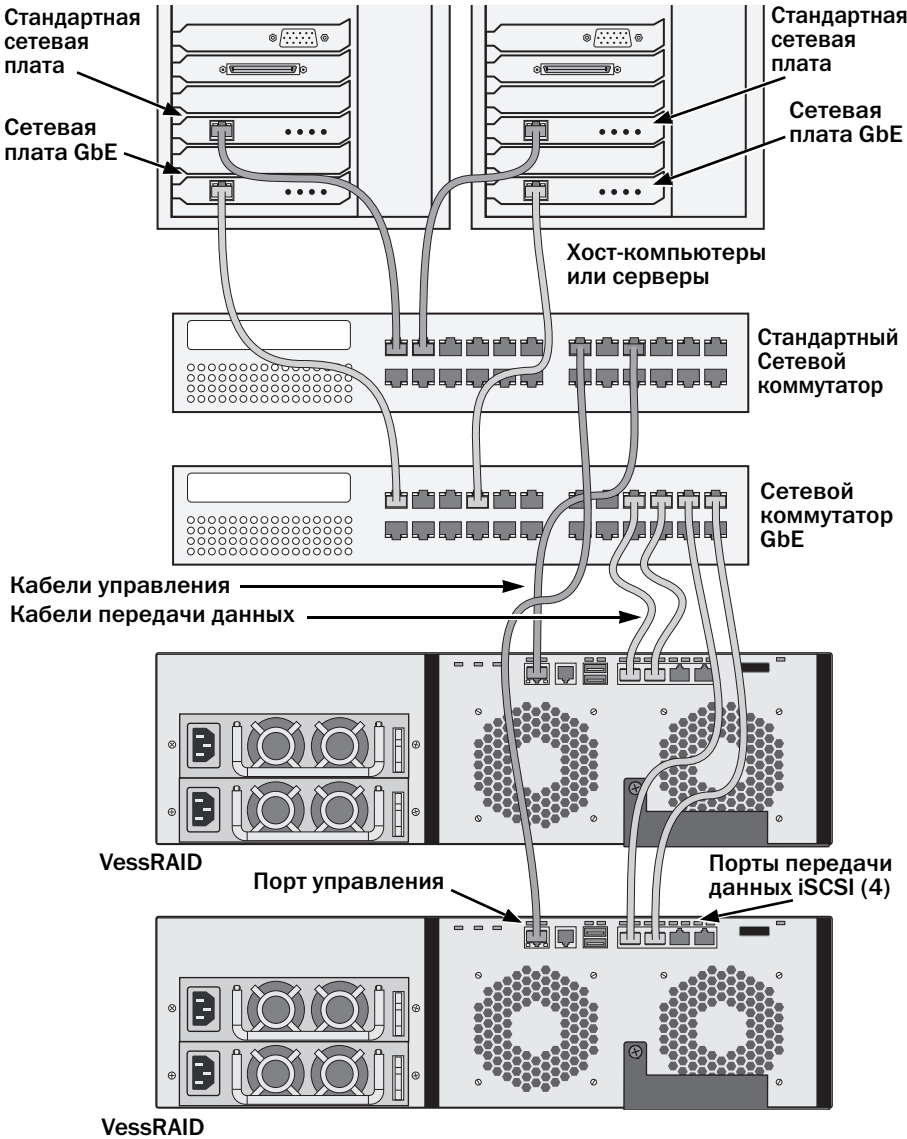
Рис. 20. Соединения для передачи данных и управления в конфигурации SAN iSCSI
