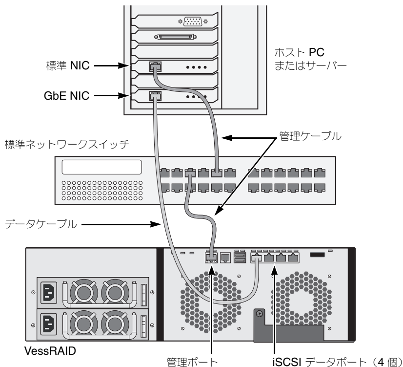
図 19. iSCSI DAS データおよび管理接続
