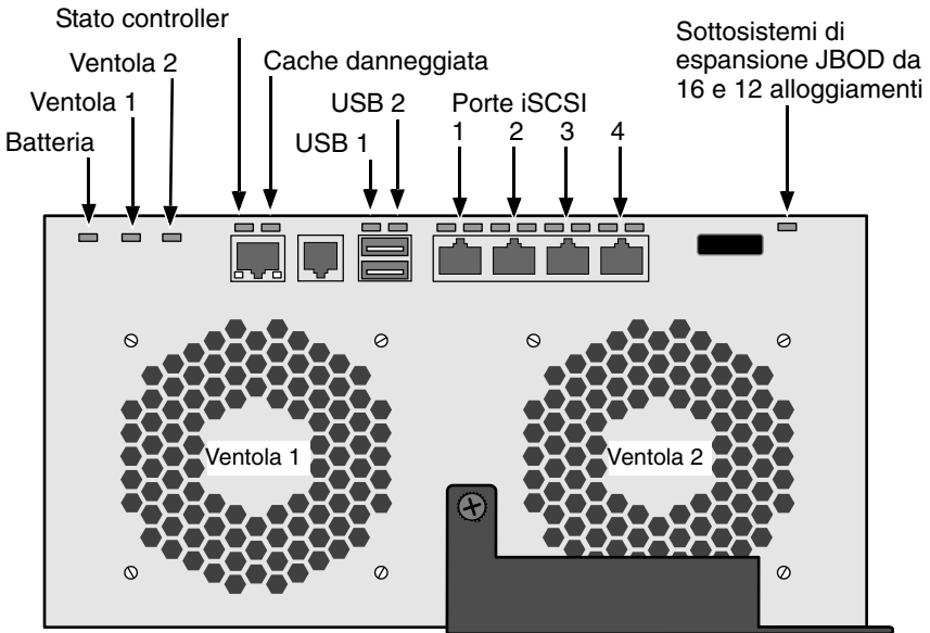
Figura 27. LED del controller iSCSI del VessRAID
