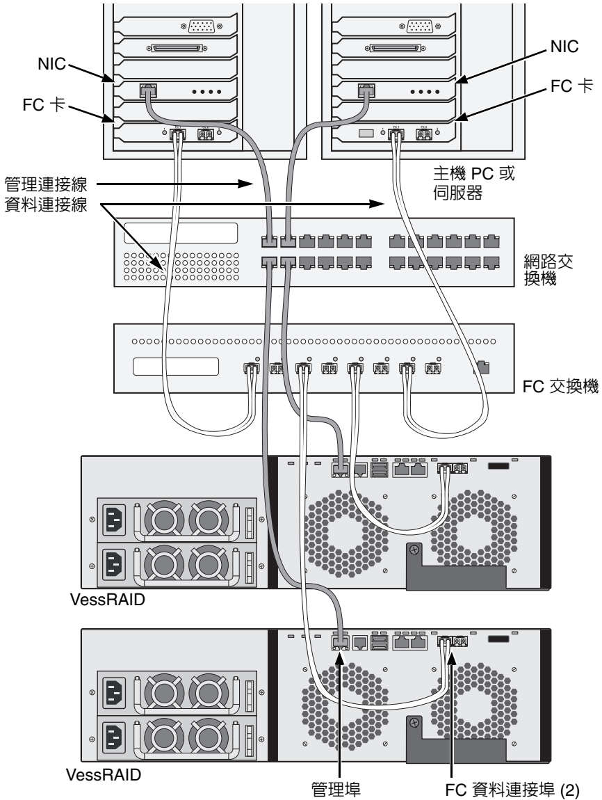
圖 17. FC SAN 資料與管理連線
