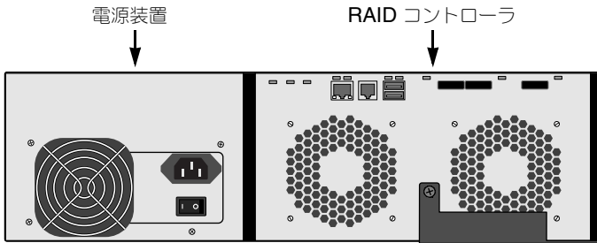
図 6. VessRAID 1740s 背面図
