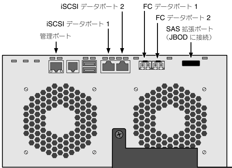
図 15. VessRAID FC データおよび管理ポート
