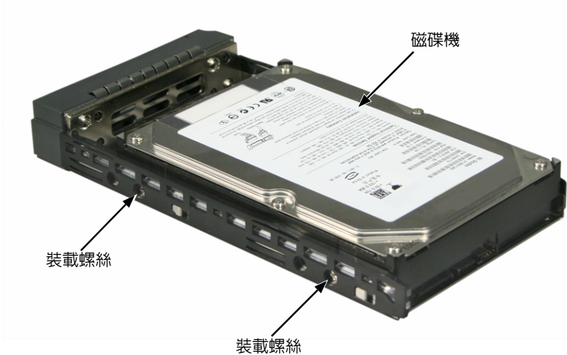
圖 14. 裝載於硬碟抽取匣內的磁碟機
