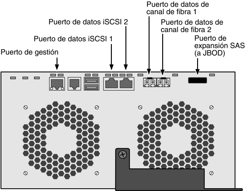
Ilustración 15. Puertos de gestión y de datos de canal de fibra de VessRAID
