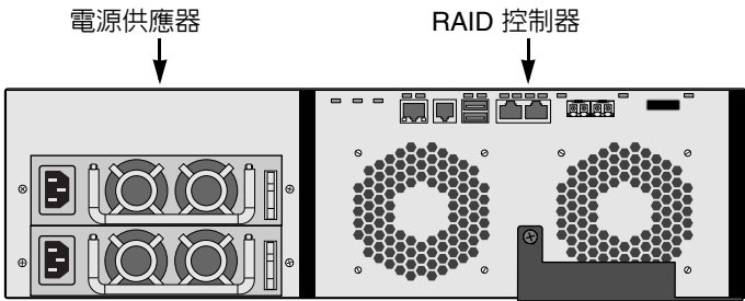
圖 2. VessRAID 1840f 後視圖
