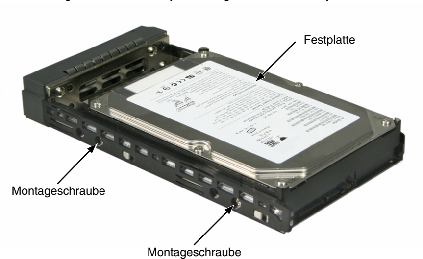
Abbildung 14. In einem Festplattenträger montierte Festplatte
