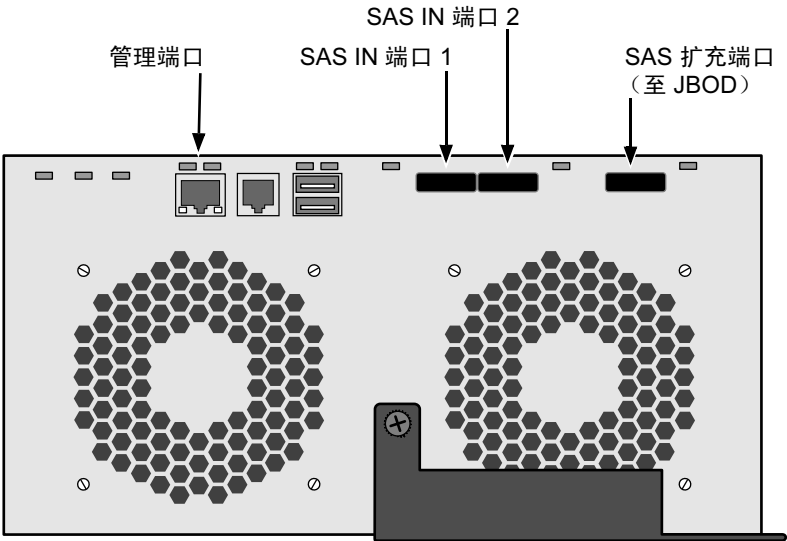
图 22。SAS DAS 数据和管理连接
