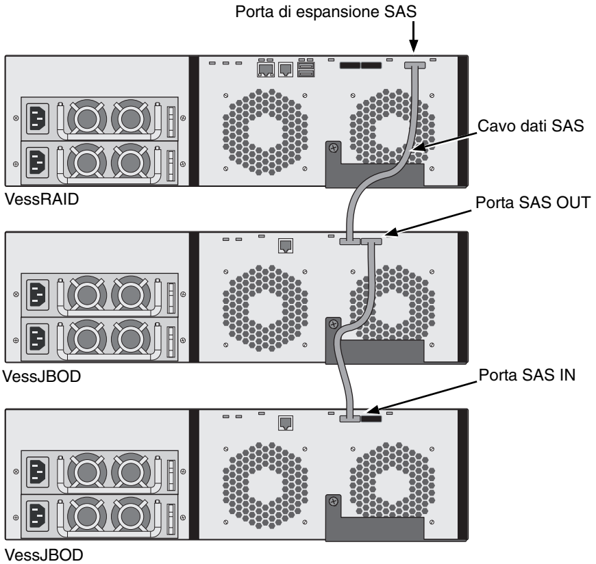
Figura 23. Collegamenti dati di espansione JBOD SAS
