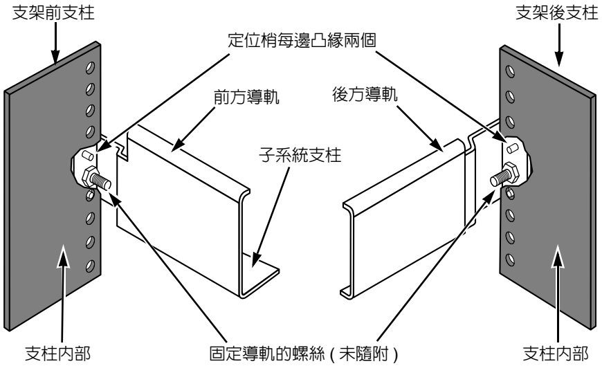
圖 10. 支架底座組件圖示
