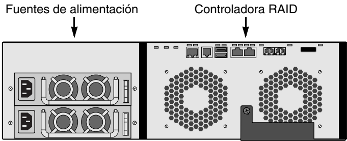
Ilustración 3. Vista posterior de la unidad VessRAID 1840i
