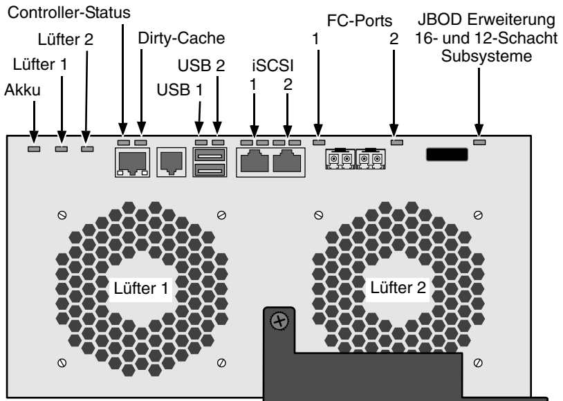
Abbildung 26. VessRAID FC-Controller-LED-Anzeigen
