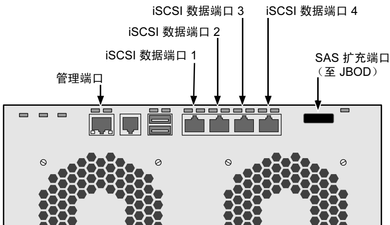
图 19。iSCSI DAS 数据和管理连接
