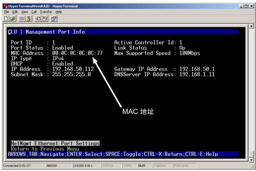
图 31。查看管理端口的 MAC 地址。
