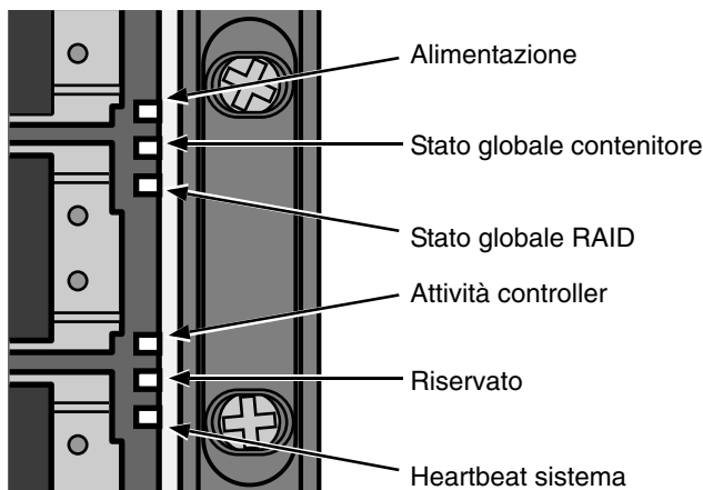
Figura 25. Visualizzazione dei LED del pannello anteriore del VessRAID
