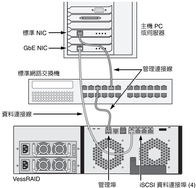
圖 19. iSCSI DAS 資料與管理連接
