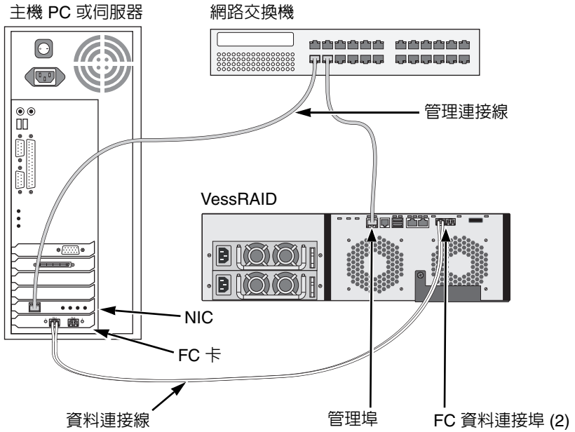
圖 16. FC DAS 資料與管理連線
