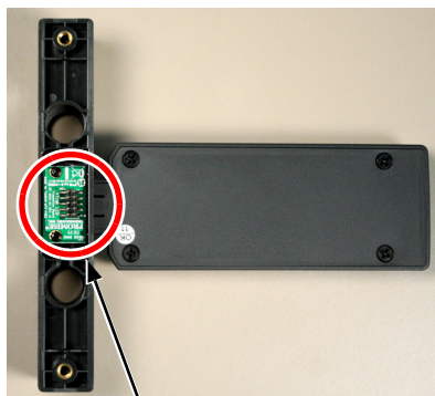
그림 7. 격납장치와 LCD 패널에 있는 커넥터를 맞추기
