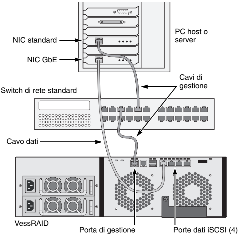
Figura 19. Collegamenti dati e gestione DAS iSCSI
