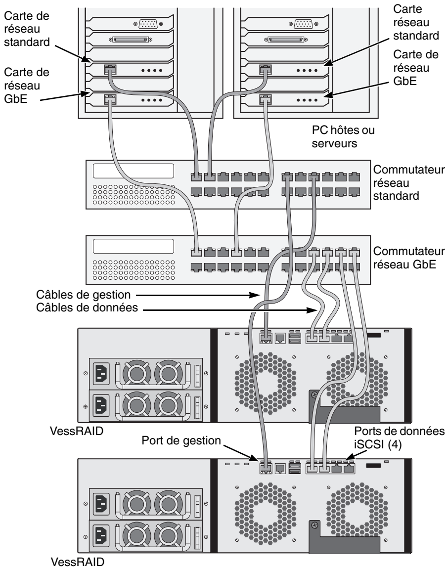
Figure 20. Connexions de gestion et de données iSCSI SAN.
