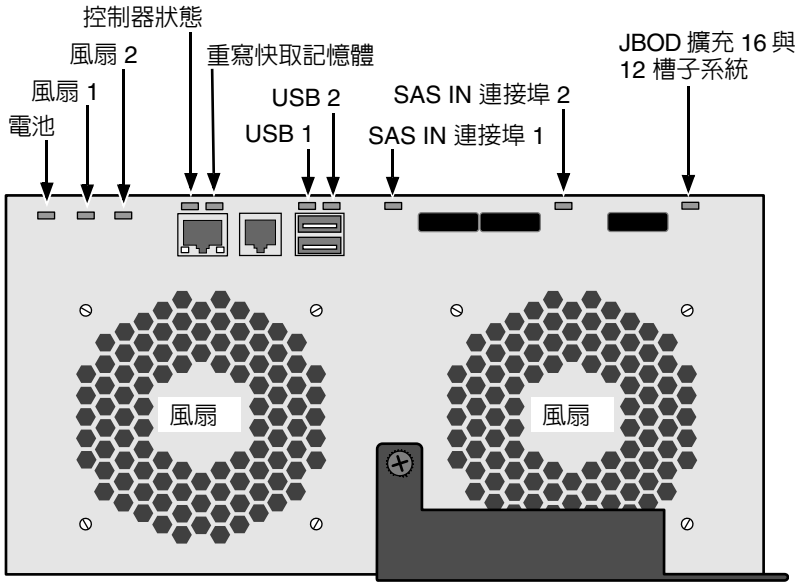
圖 28. VessRAID SAS 控制器 LED
