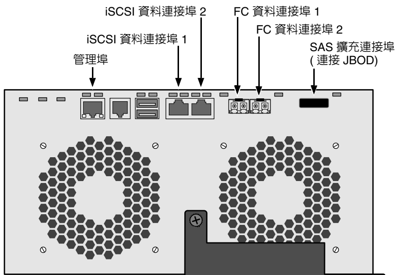
圖 15. VessRAID FC 資料與管理連接埠
