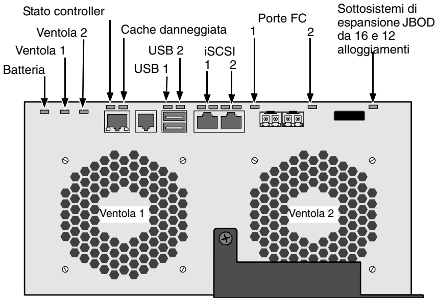
Figura 26. LED del controller FC del VessRAID
