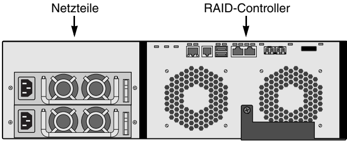
Abbildung 3. VessRAID 1840i Rückansicht
