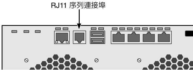
圖 24. 序列連接埠位於控制器上
