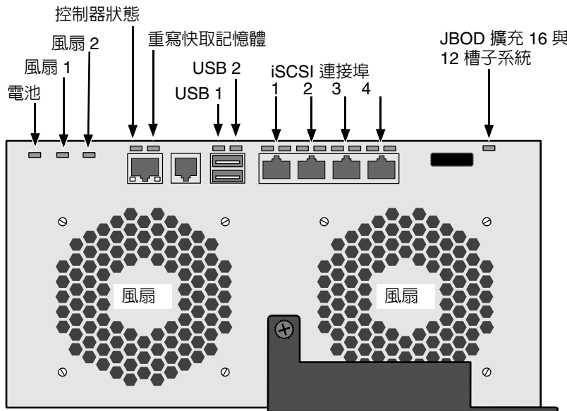
圖 27. VessRAID iSCSI 控制器 LED
