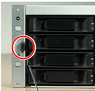
그림 7. 격납장치와 LCD 패널에 있는 커넥터를 맞추기
