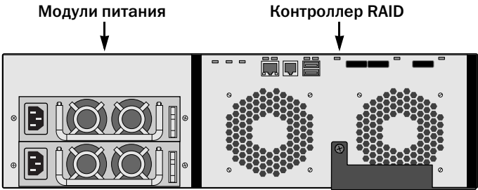
Рис. 5. Вид устройства VessRAID 1740i сзади
