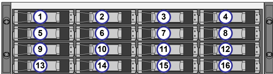
Abbildung 11. Nummerierung der 16-Schacht VessRAID-Laufwerkssteckplätze
