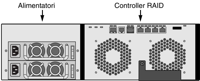
Figura 4. Vista posteriore del VessRAID 1840s
