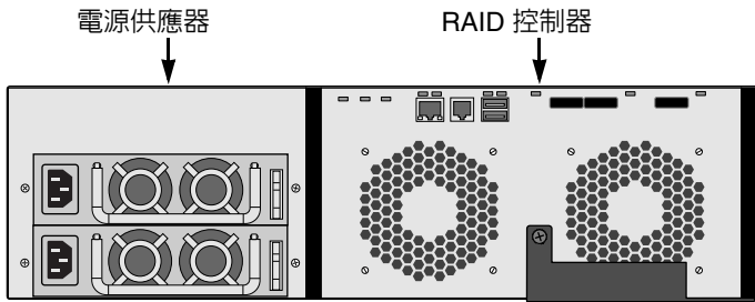
圖 5. VessRAID 1740i 後視圖
