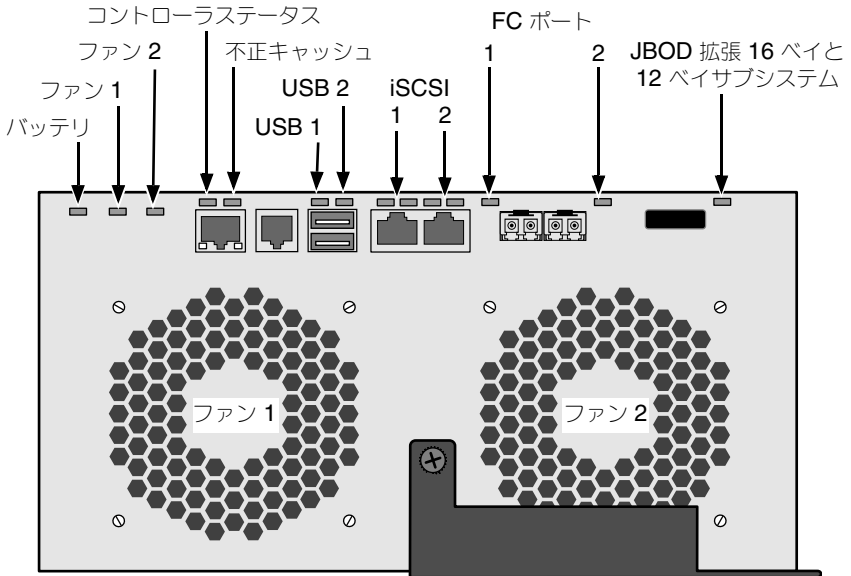
図 26. VessRAID FC コントローラ LED
