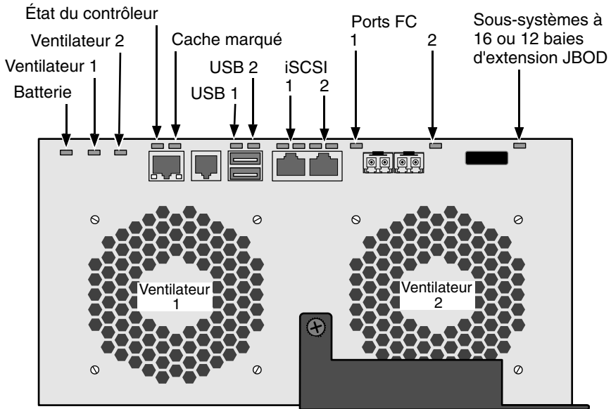
Figure 26. Voyants du contrôleur VessRAID
