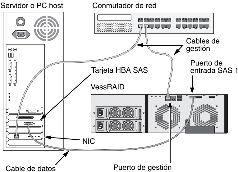
Ilustración 22. Conexiones de gestión y datos de DAS SAS
