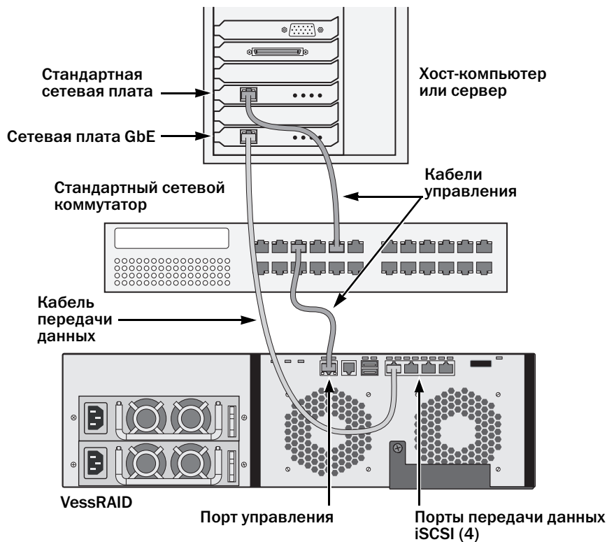
Рис. 19. Соединения для передачи данных и управления в конфигурации DAS iSCSI
