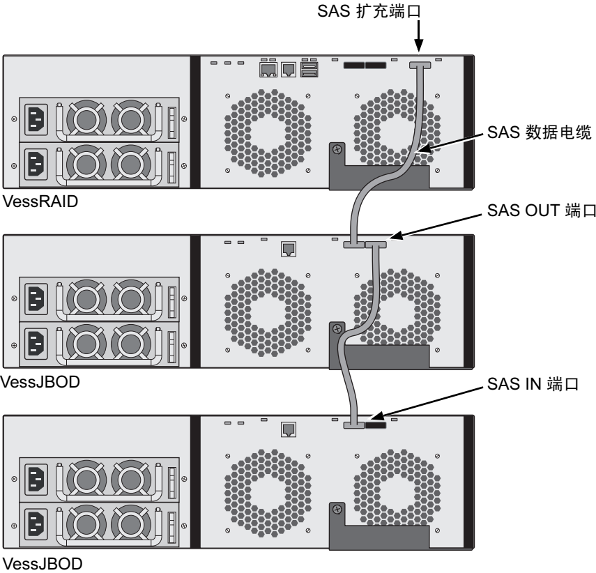
图 23。SAS JBOD 扩充数据连接
