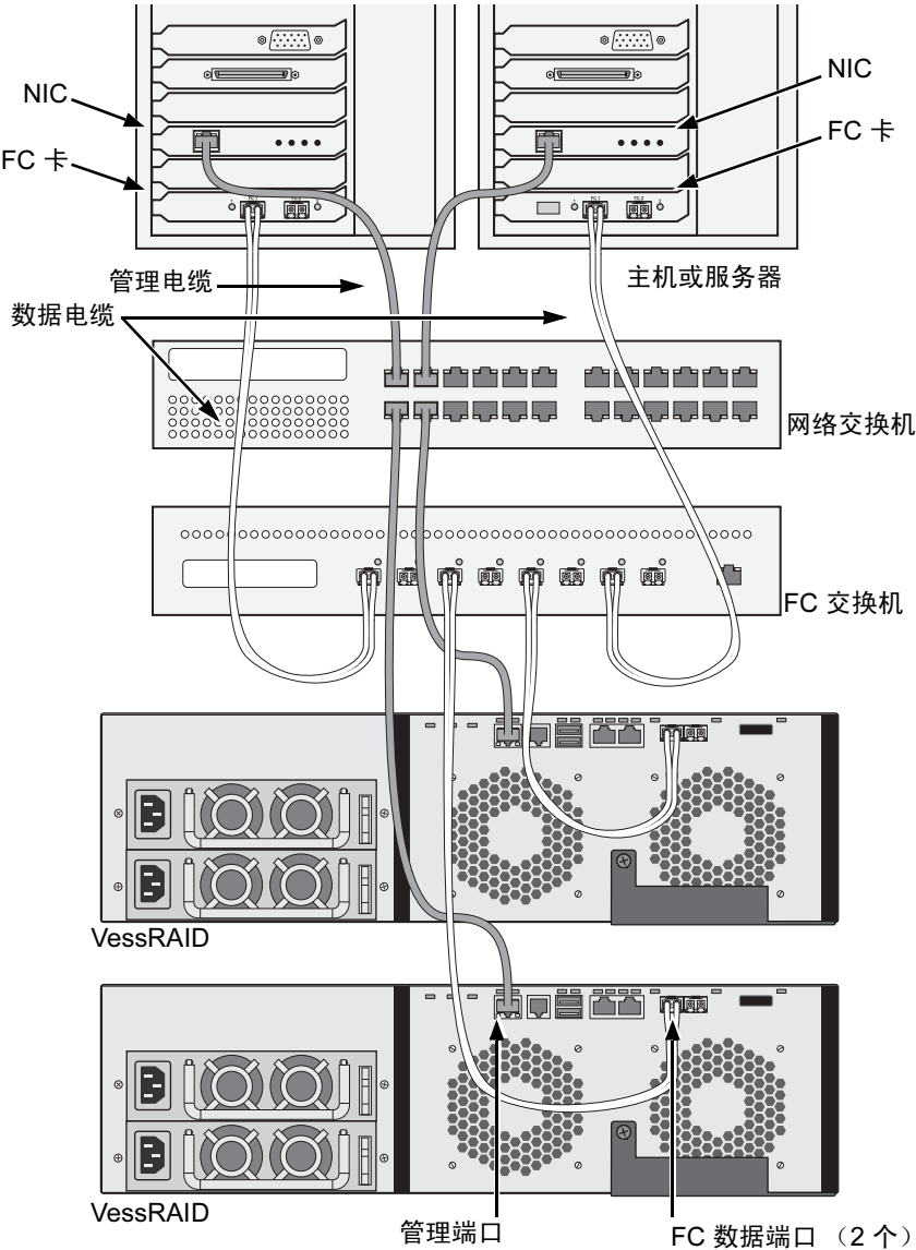
图 17。FC SAN 数据和管理连接
