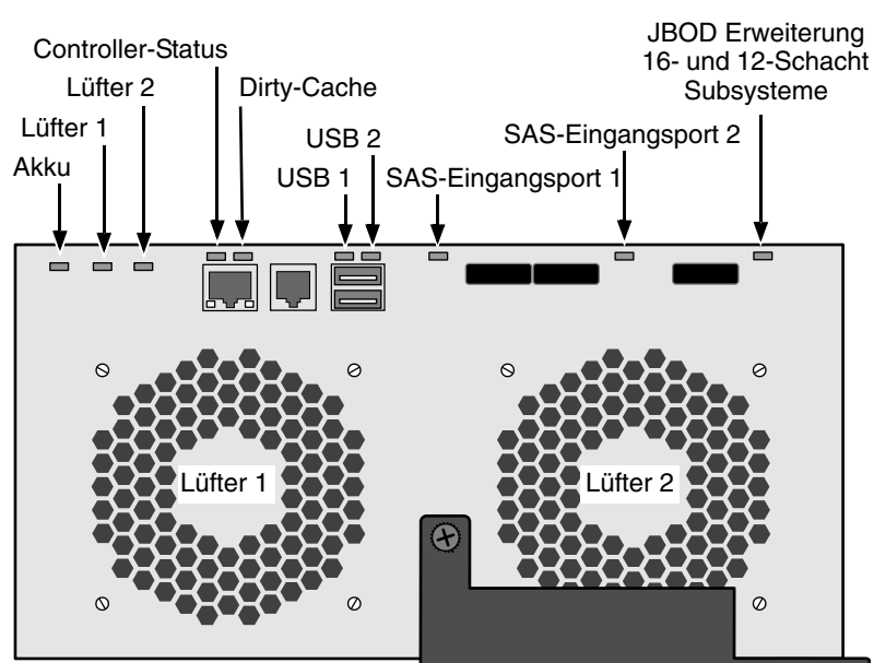
Abbildung 28. VessRAID SAS-Controller-LED-Anzeigen
