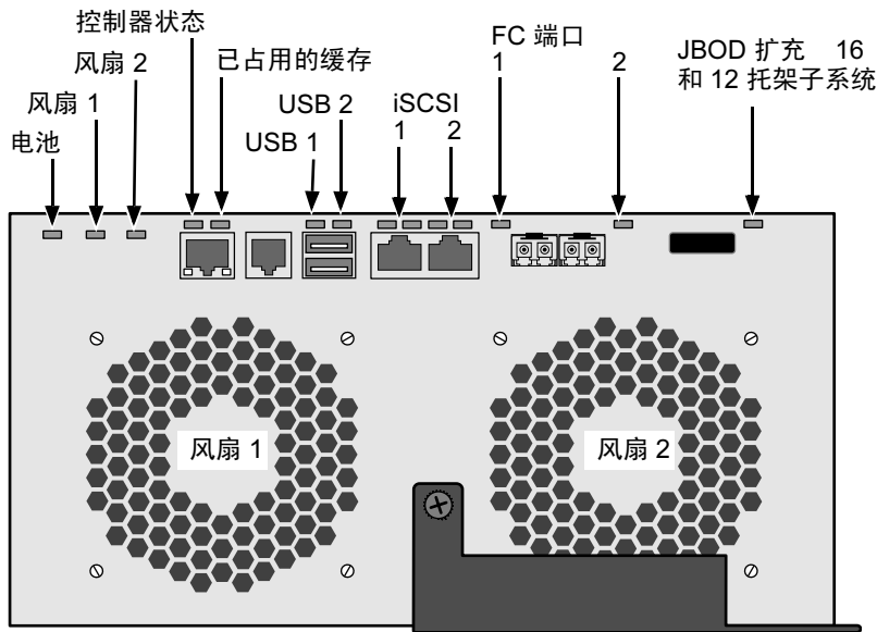
图 26。VessRAID FC 控制器 LED 指示灯
