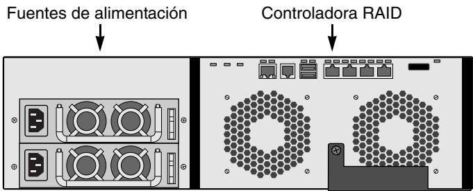
Ilustración 4. Vista posterior de la unidad VessRAID 1840s
