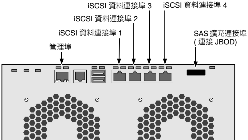
圖 19. iSCSI DAS 資料與管理連接
