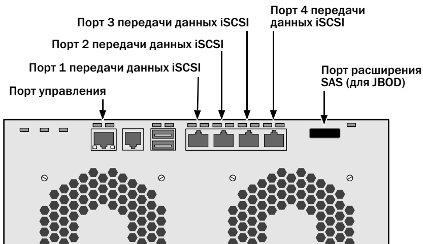
Рис. 18. Порты передачи данных и управления iSCSI устройства VessRAID
