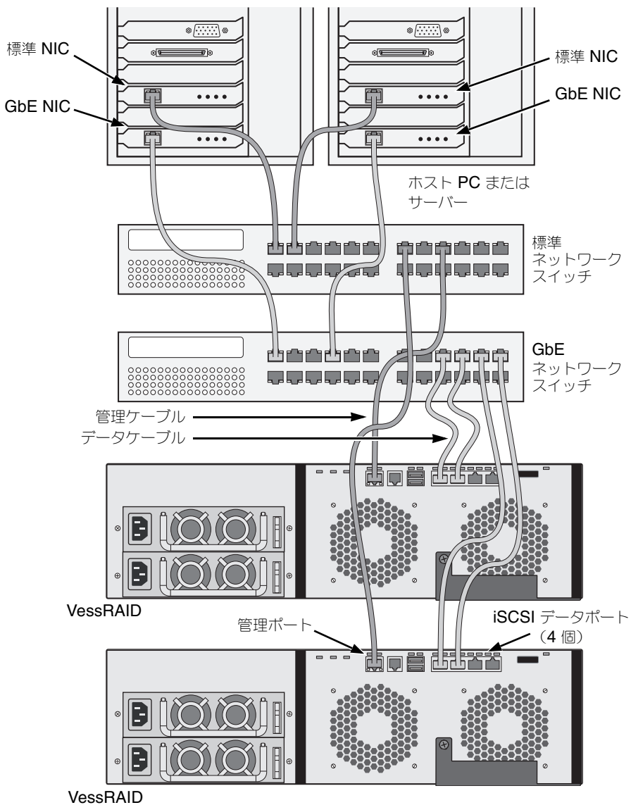
図 20. iSCSI SAN データおよび管理接続
