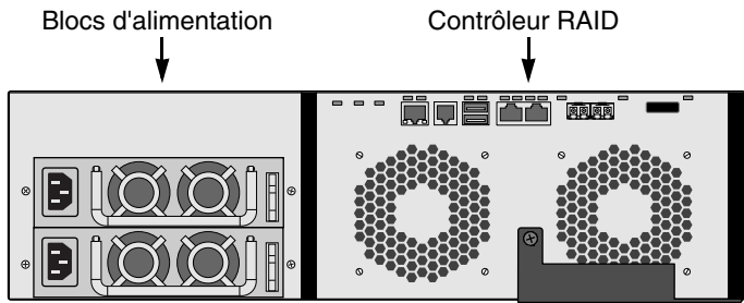
Figure 3. Vue arrière du VessRAID 1840i
