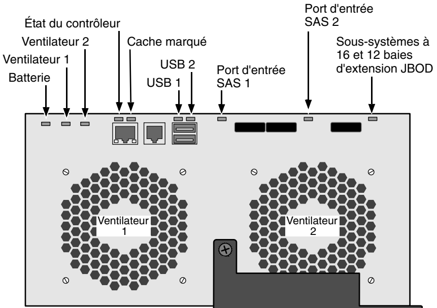
Figure 28. Voyants du contrôleur SAS VessRAID
