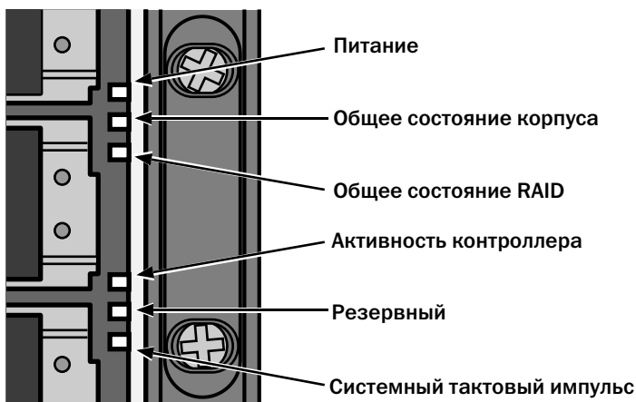
Рис. 25. Индикаторы на передней панели устройства VessRAID
