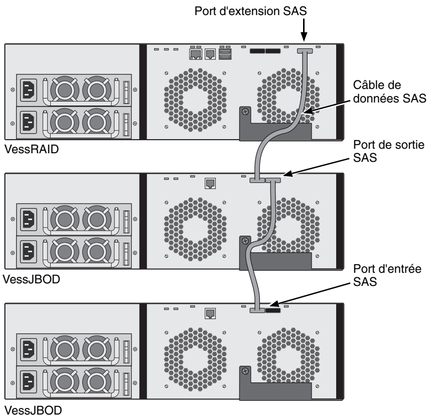
Figure 23. Connexions de données d'extension JBOD SAS
