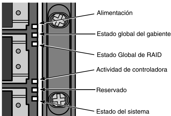
Ilustración 25. Pantalla LED del panel anterior de la unidad VessRAID
