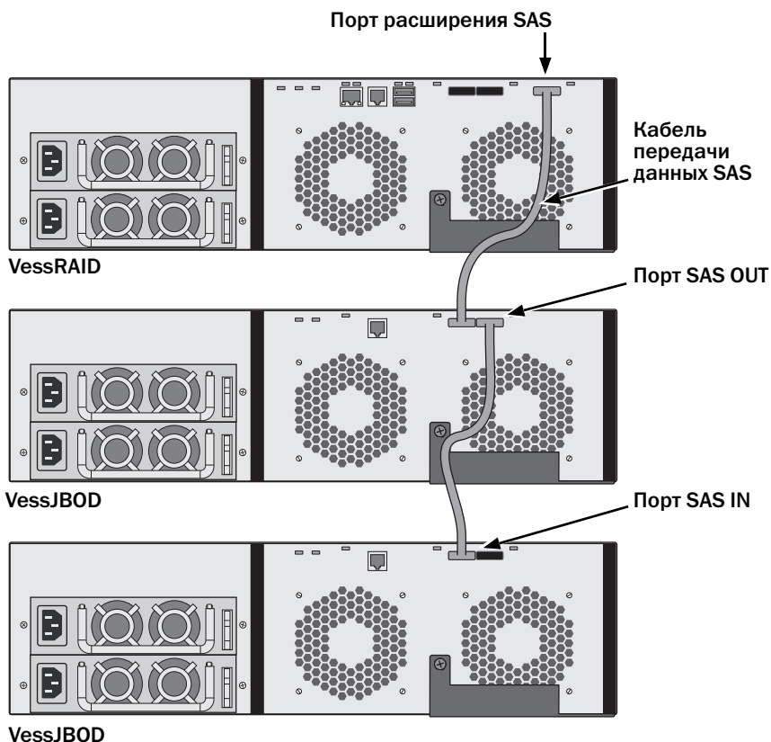
Рис. 23. Соединения для передачи данных расширения SAS JBOD
