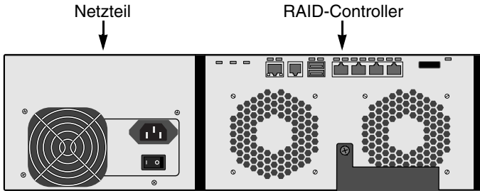
Abbildung 6. VessRAID 1740s Rückansicht
