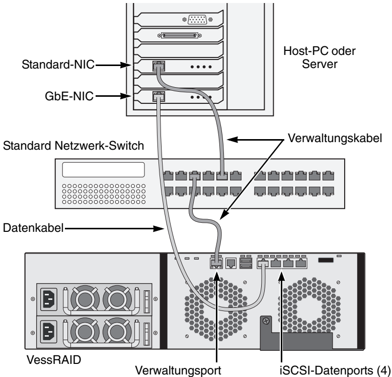
Abbildung 19. iSCSI DAS-Daten- und Verwaltungsanschlüsse
