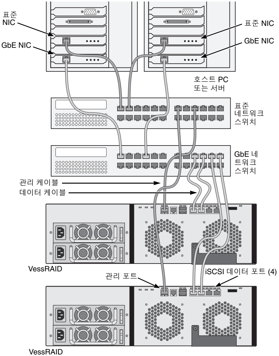
그림 20. iSCSI SAN 데이터 및 관리 연결
