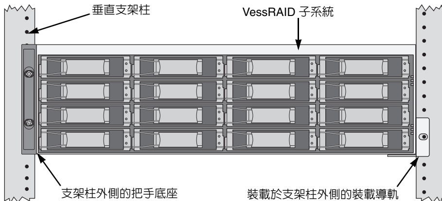
圖 9. 安裝在可用導軌支架中的 16 槽 VessRAID
