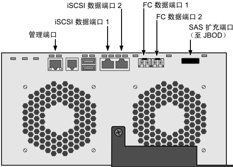
图 15。 VessRAID FC 数据和管理端口
