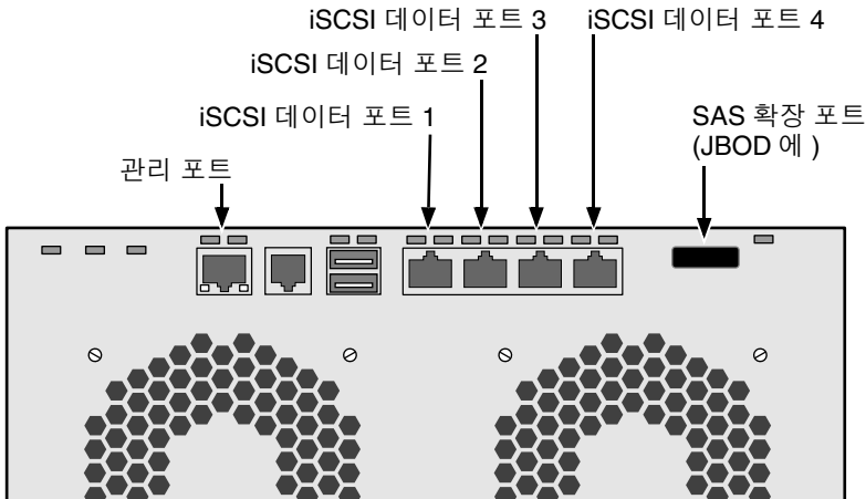
그림 18. VessRAID iSCSI 데이터 및 관리 포트
