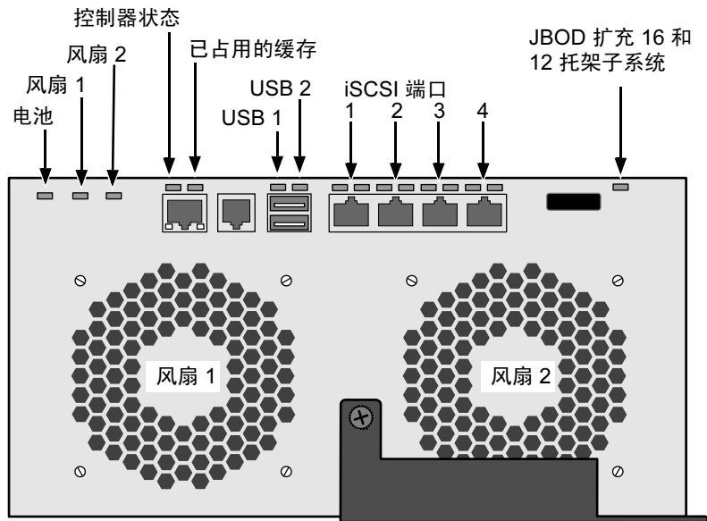
图 27。VessRAID iSCSI 控制器 LED 指示灯
