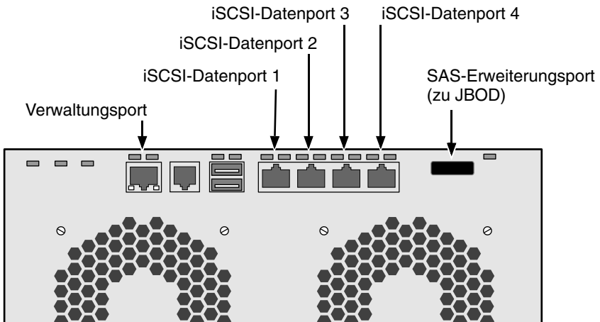
Abbildung 19. iSCSI DAS-Daten- und Verwaltungsanschlüsse
