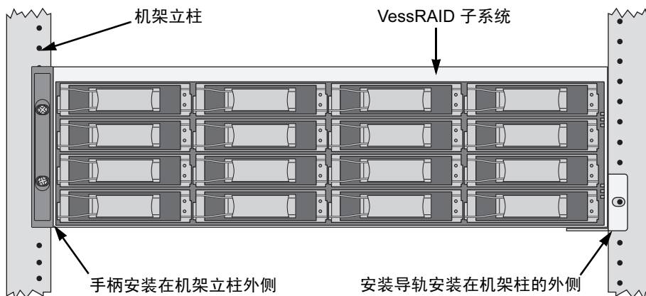
图 9. 安装到机架中的 16 托架 VessRAID，带有可用的导轨
