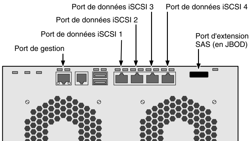
Figure 19. Connexions de gestion et de données iSCSI DAS
