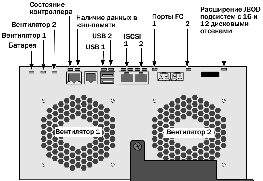
Рис. 26. Индикаторы контроллера VessRAID FC
