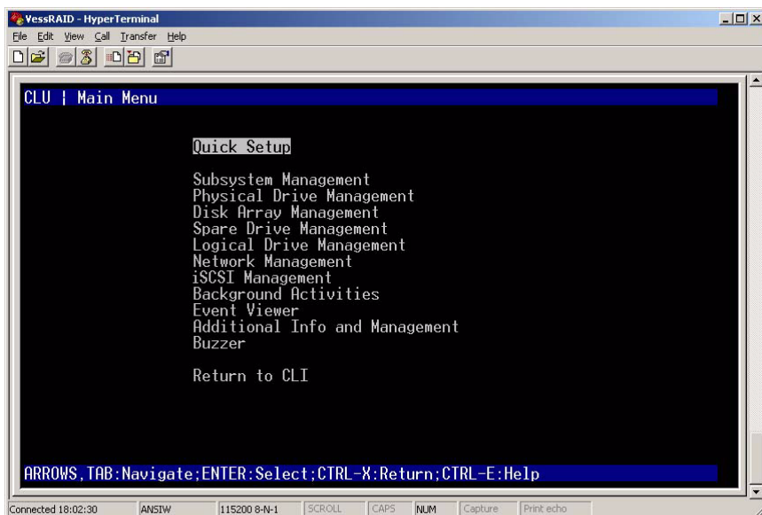
Рис. 32. Главное меню утилиты командной строки
