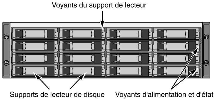
Figure 1. Vue frontale du VessRAID à 16 baies
