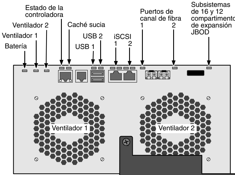
Ilustración 26. LED de la controladora de canal de fibra la unidad VessRAID
