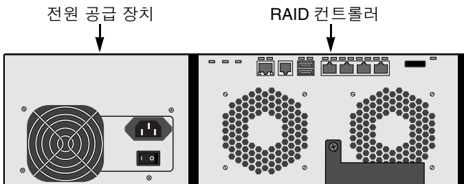
그림 5. VessRAID 1740i 후면 모습
