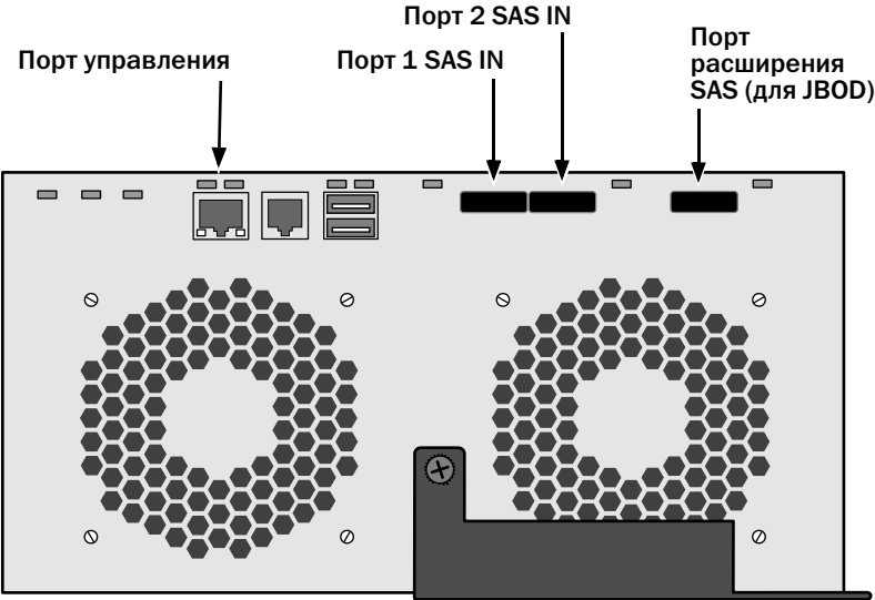
Рис. 22. Соединения для передачи данных и управления в конфигурации DAS SAS
