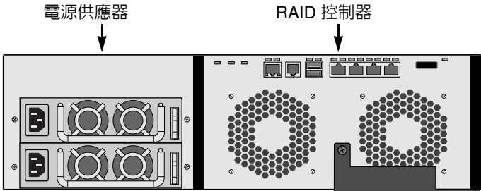
圖 4. VessRAID 1840s 後視圖
