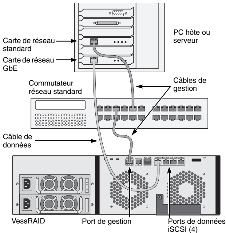
Figure 19. Connexions de gestion et de données iSCSI DAS
