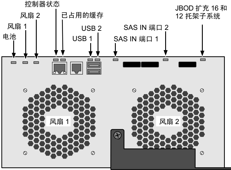
图 28。VessRAID SAS 控制器 LED 指示灯
