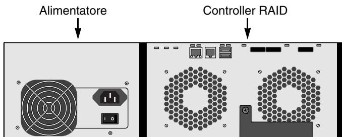
Figura 6. Vista posteriore del VessRAID 1740s
