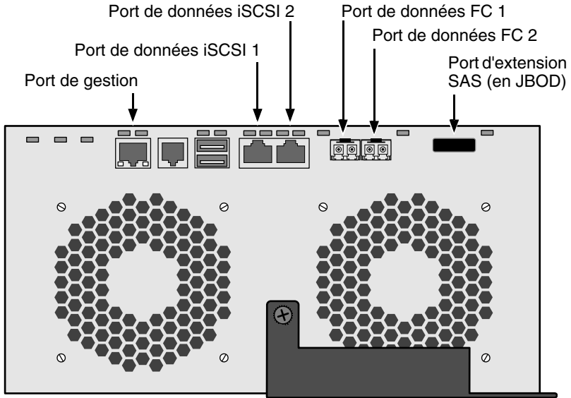
Figure 16. Connexions de gestion et de données FC DAS
