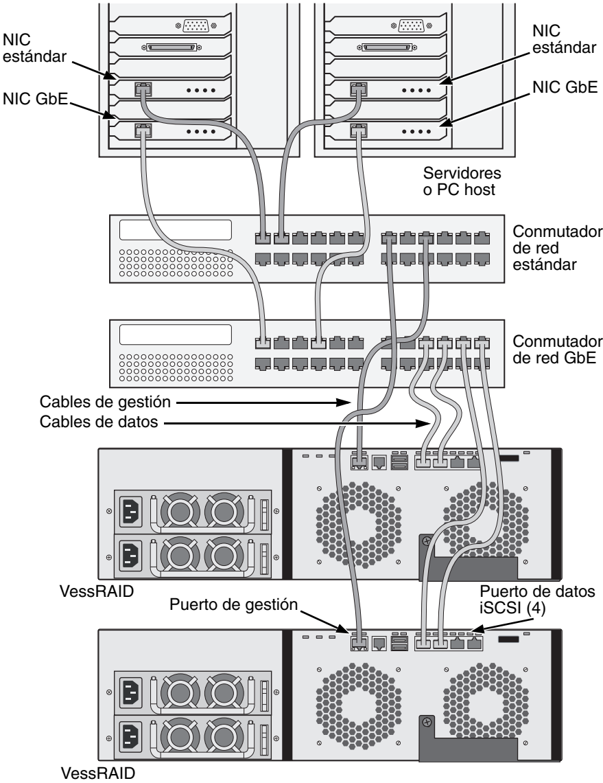
Ilustración 20. Conexiones de gestión y datos de SAN iSCSI
