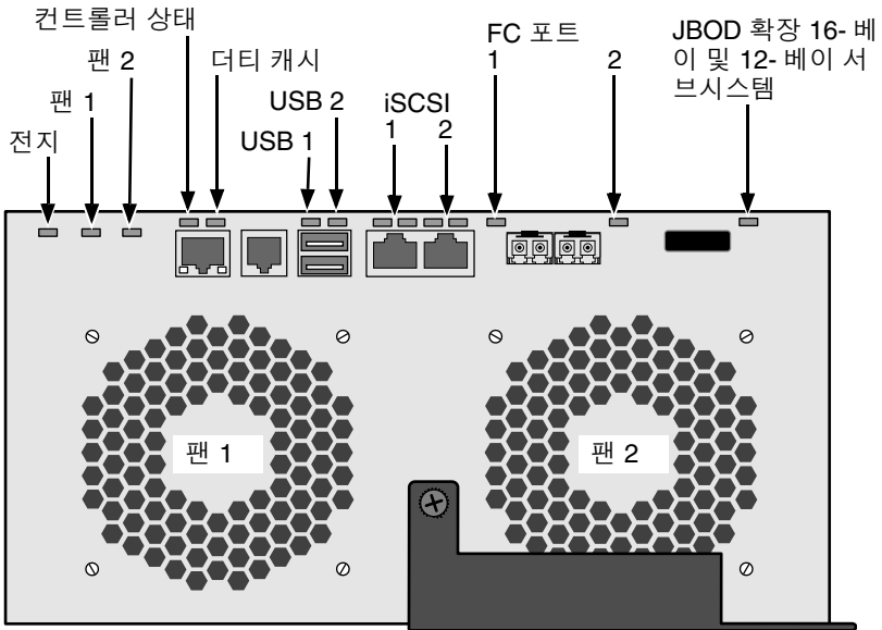
그림 26. VessRAID FC 컨트롤러 LEDs
