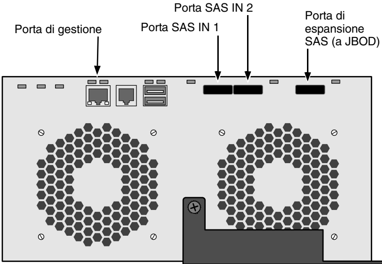
Figura 22. Collegamenti dati e gestione DAS SAS
