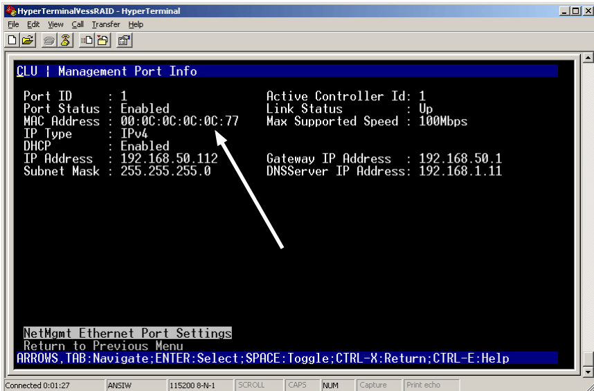
Figure 31. Affichage de l'adresse MAC du port de gestion
