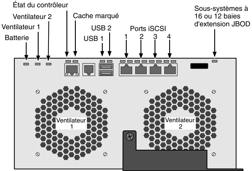
Figure 27. Voyants du contrôleur iSCSI VessRAID
