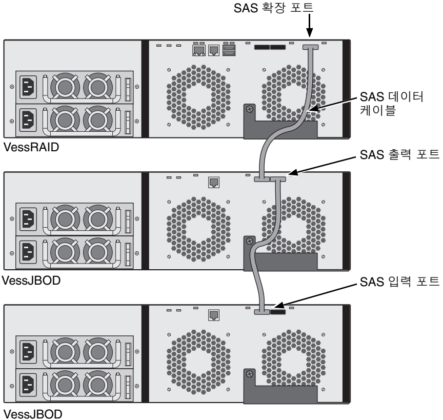
그림 23. SAS JBOD 확장 데이터 연결
