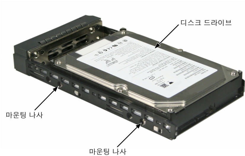
그림 14. 드라이브 캐리어에 설치된 디스크 드라이브
