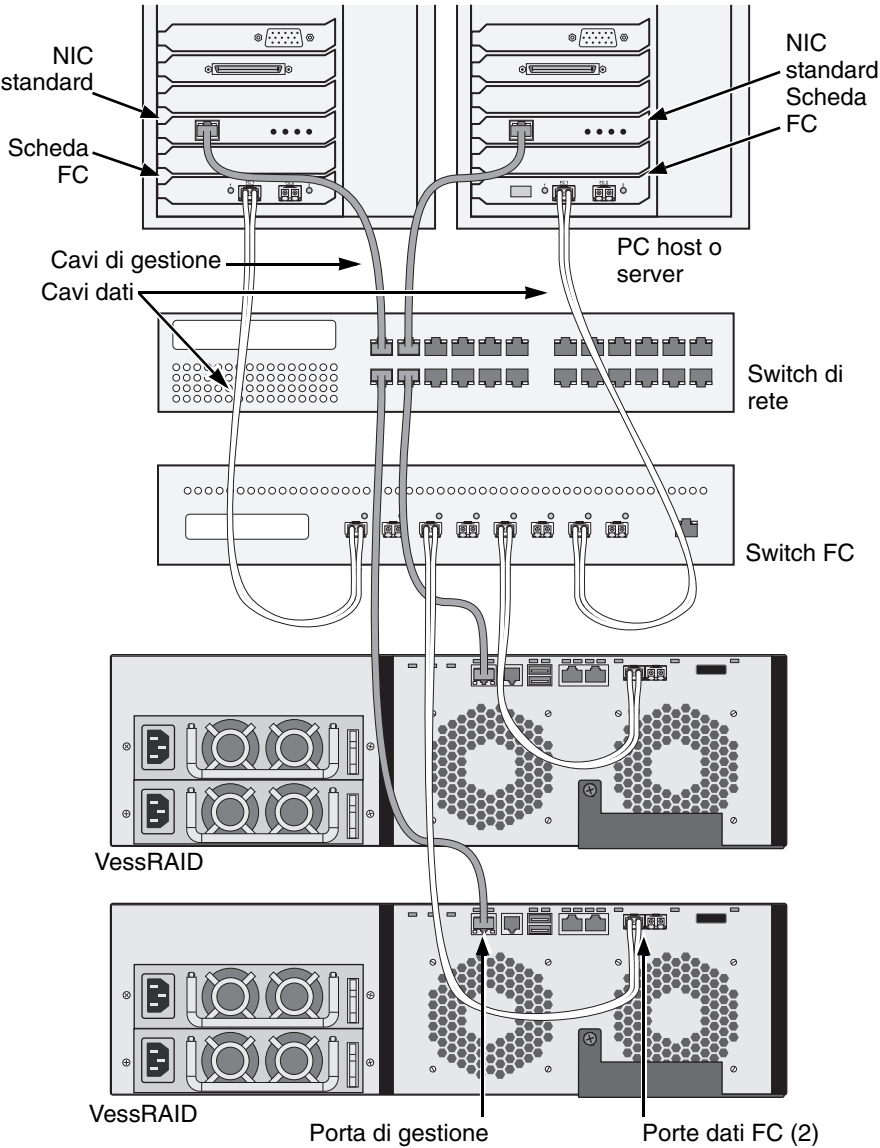
Figura 17. Collegamenti dati e gestione SAN FC
