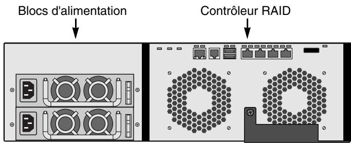
Figure 4. Vue arrière du VessRAID 1840s
