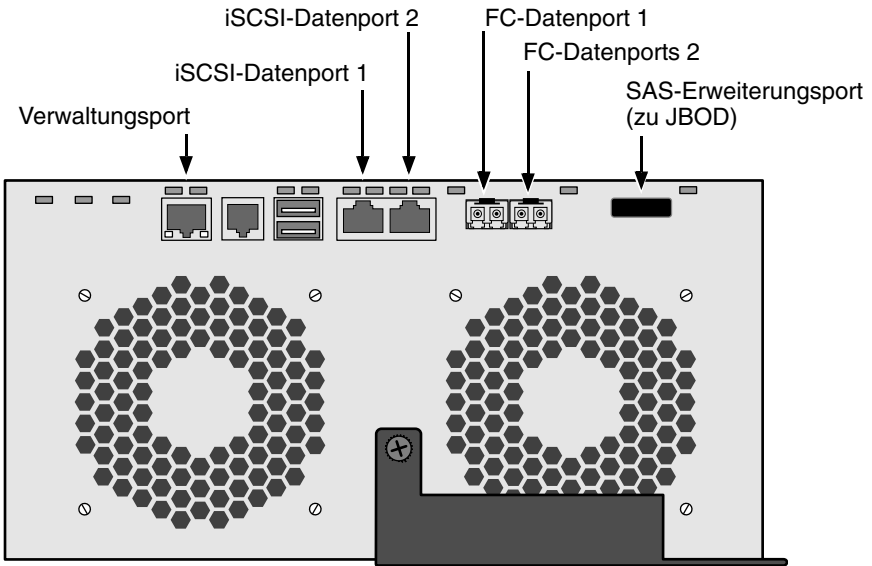
Abbildung 16. FC DAS-Daten- und Verwaltungsanschlüsse
