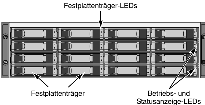
Abbildung 1. 16-Schacht VessRAID Vorderansicht
