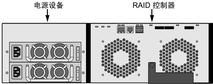
图 5. VessRAID 1740i 后视图
