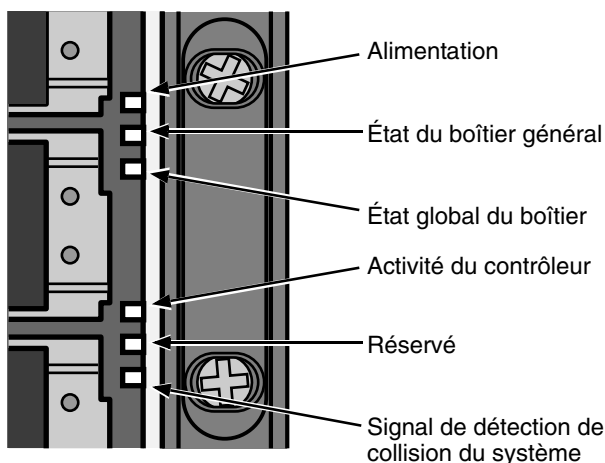
Figure 25. DEL du panneau avant du VessRAID
