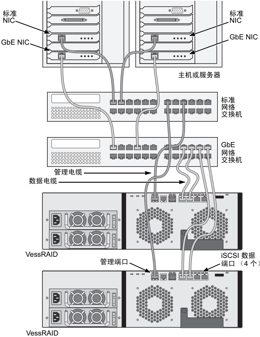
图 20。iSCSI SAN 数据和管理连接
