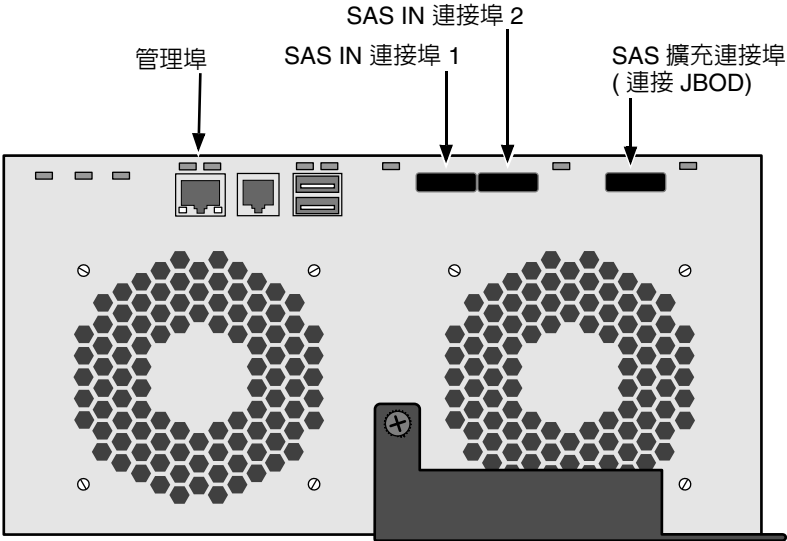
圖 22. SAS DAS 資料與管理連接
