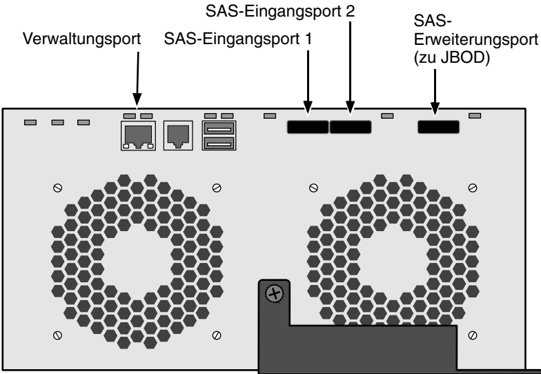
Abbildung 22. SAS DAS-Daten- und Verwaltungsanschlüsse
