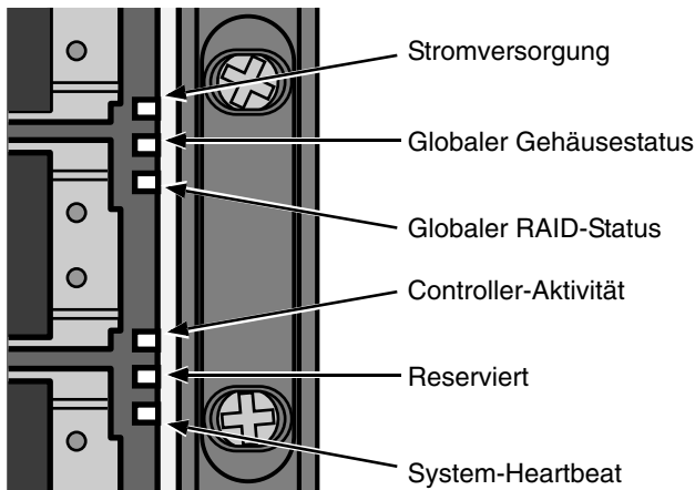
Abbildung 25. LED-Display auf der Vorderseite des VessRAID
